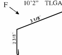
⑳ Gutter Apron 10'2" TLGA29xx
